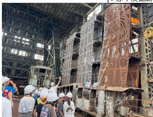
▼赤平炭鉱跡
